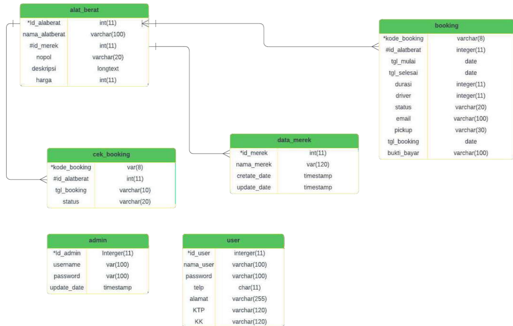
Gambar 4.8 Relasi Antar Tabel
