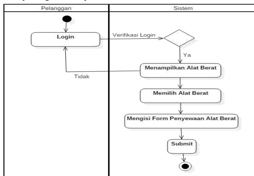
Gambar 4.4 Activity Diagram Penyewaan Alat berat
