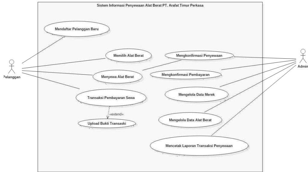
Gambar 4.2 Use Case Diagram sistem yang diusulkan
