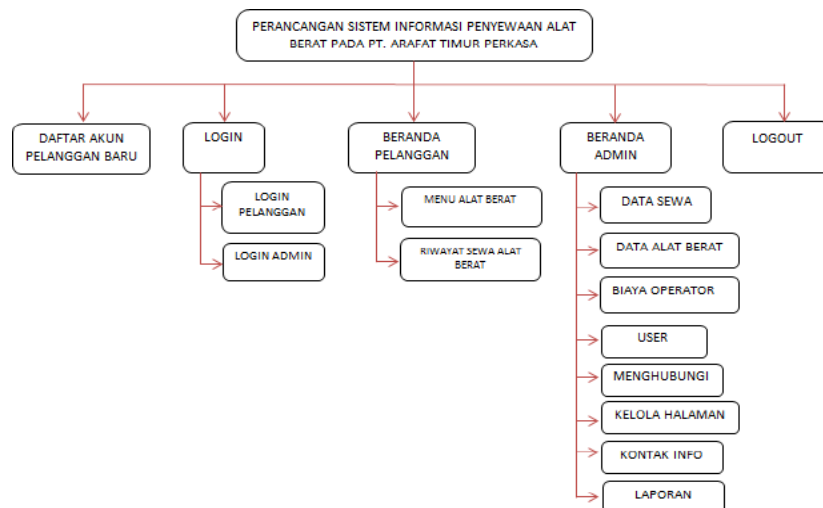
Gambar 4.9 Rancangan program secara umum
