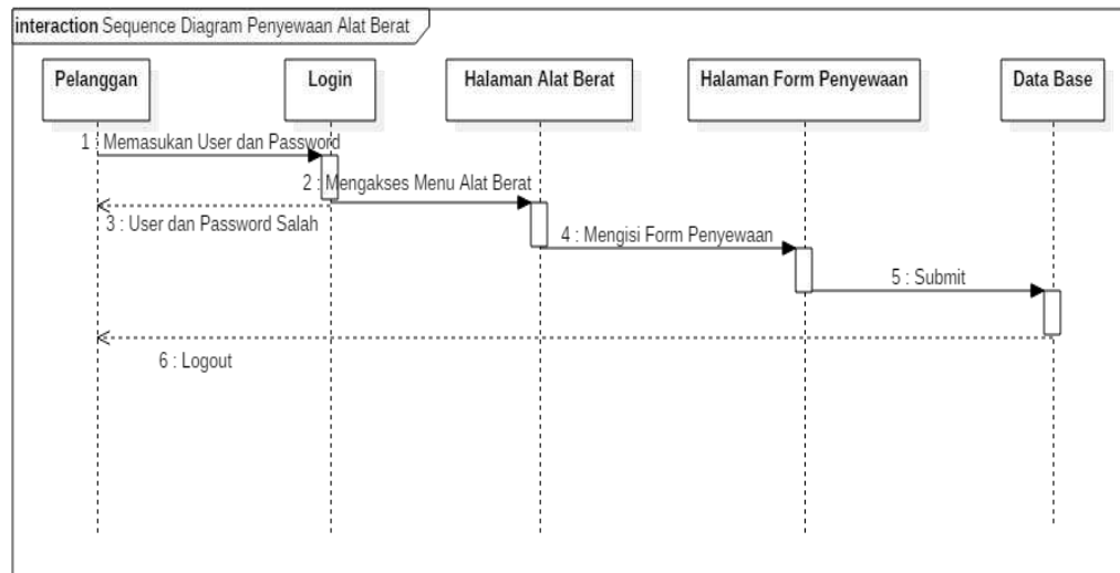
Gambar 4.7 Sequence Diagram Penyewaan Alat berat
