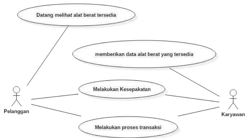
Gambar 4.1 Use Case Diagram sistem yang berjalan
