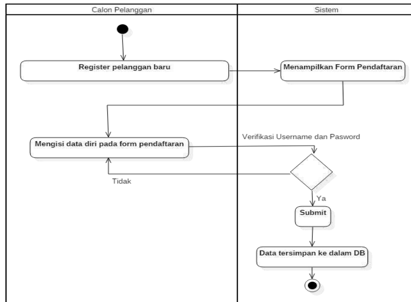
Gambar 4.3 Activity Diagram Pendaftaran Calon Pelanggan
